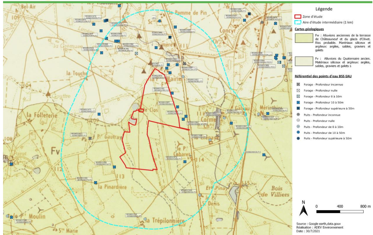
Contexte géologique
